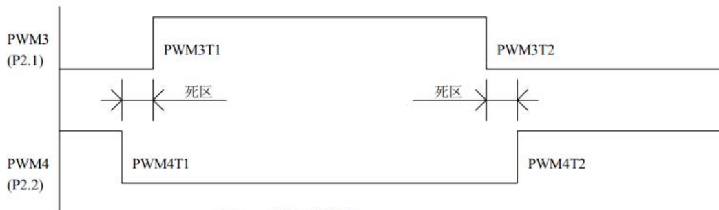
图2: 死区说明
